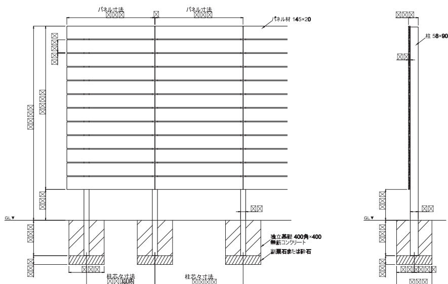
基礎図
