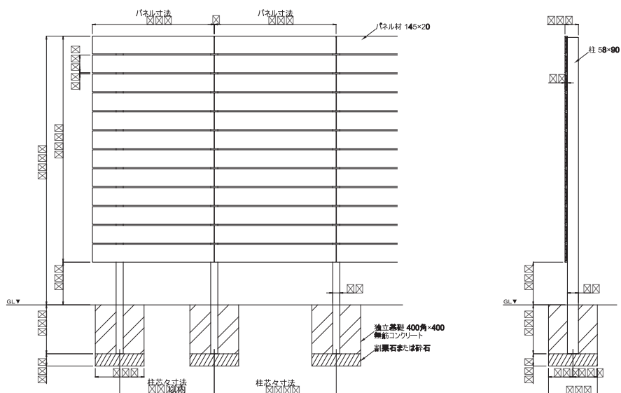
基礎図
