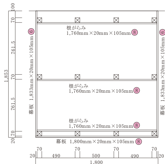
根がらみ 幕板配置図
