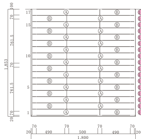
床板配置図
