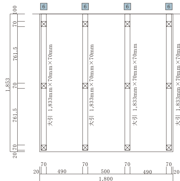
大引配置図
