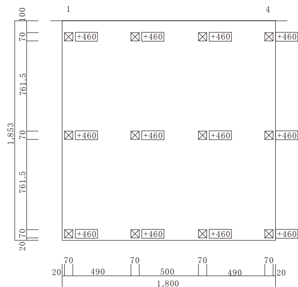
束配置図
