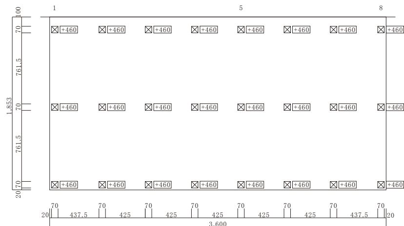
束配置図
