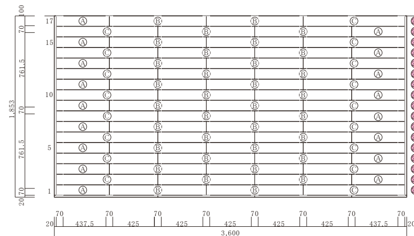
床板配置図
