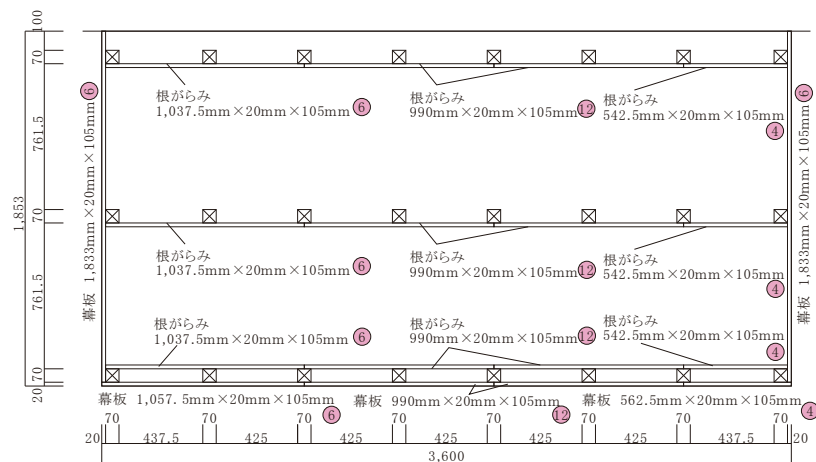
根がらみ・幕板配置図
