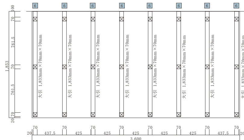
大引配置図
