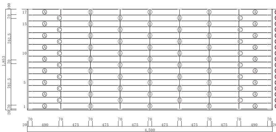
床板配置図
