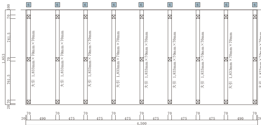
大引配置図
