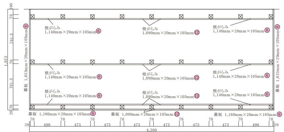
根がらみ・幕板配置図
