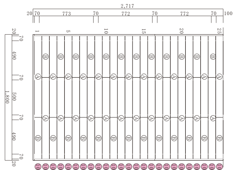
床板配置図
