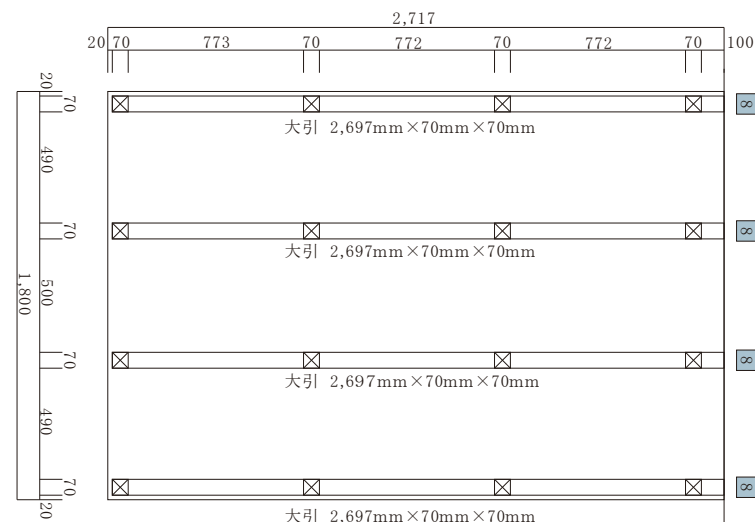
大引配置図
