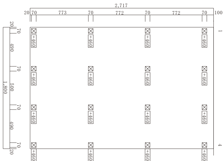
束配置図
