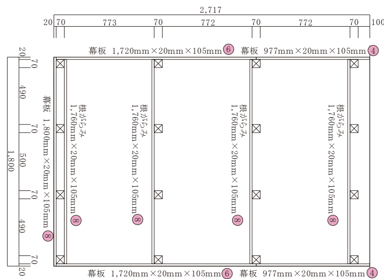
根がらみ 幕板配置図
