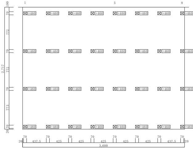
束配置図
