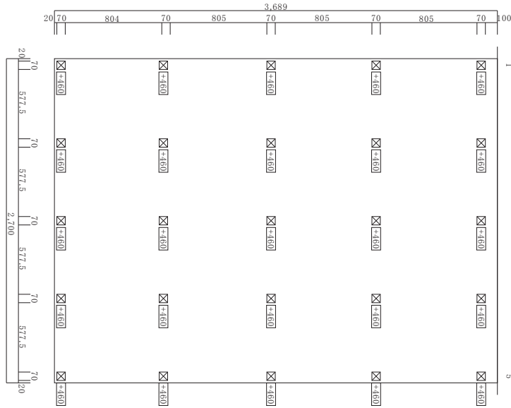
束配置図
