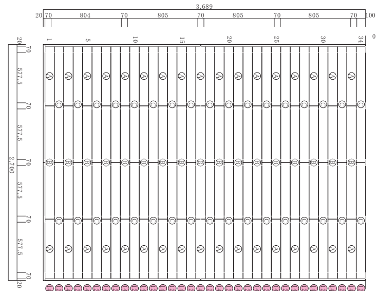
床板配置図
