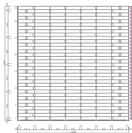
床板配置図
