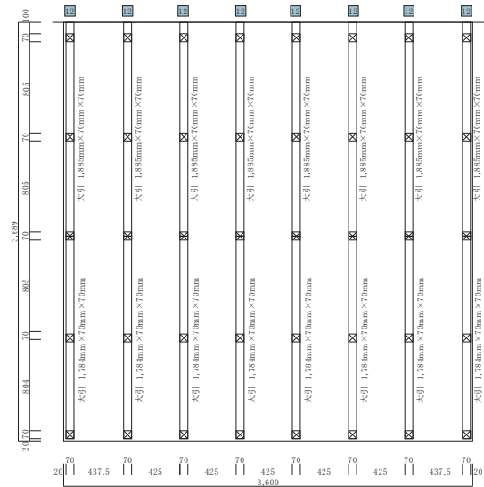
大引配置図
