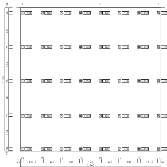
束配置図
