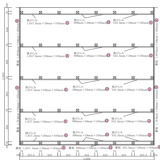
根がらみ 幕板配置図
