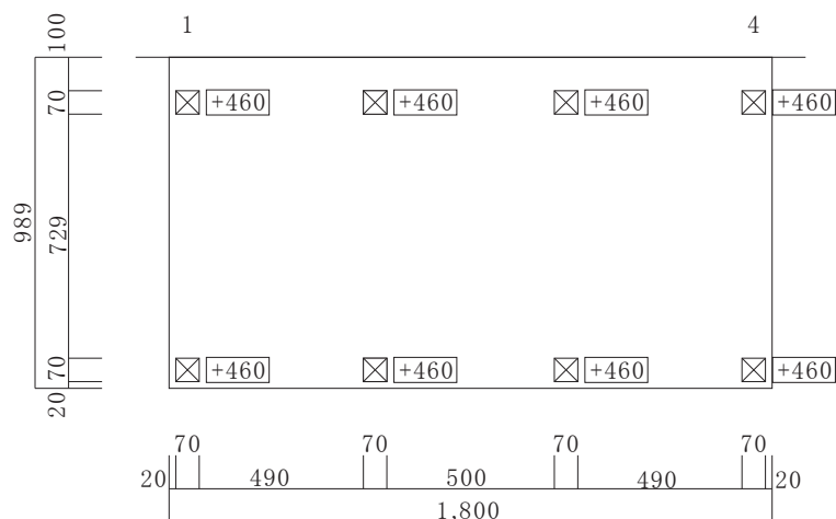
束配置図
