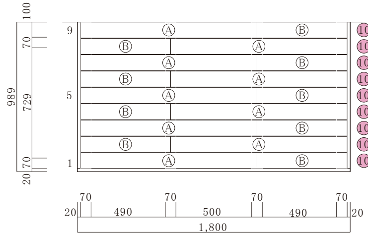
床板配置図
