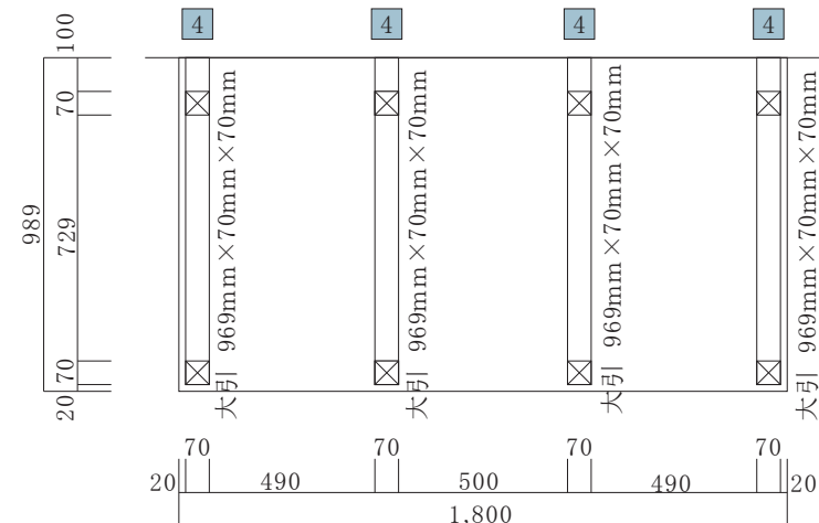
大引配置図
